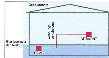
Bauweise im Einfamilien-/Zweifamilienhaus (schematische Darstellung)
