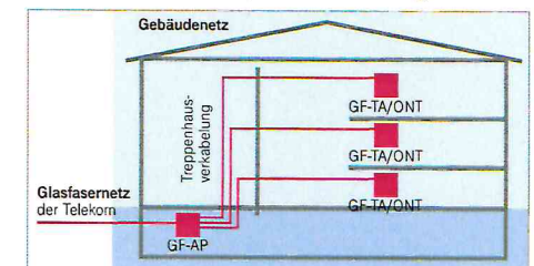
Bauweise im Mehrfamilienhaus (schematische Darstellung)
